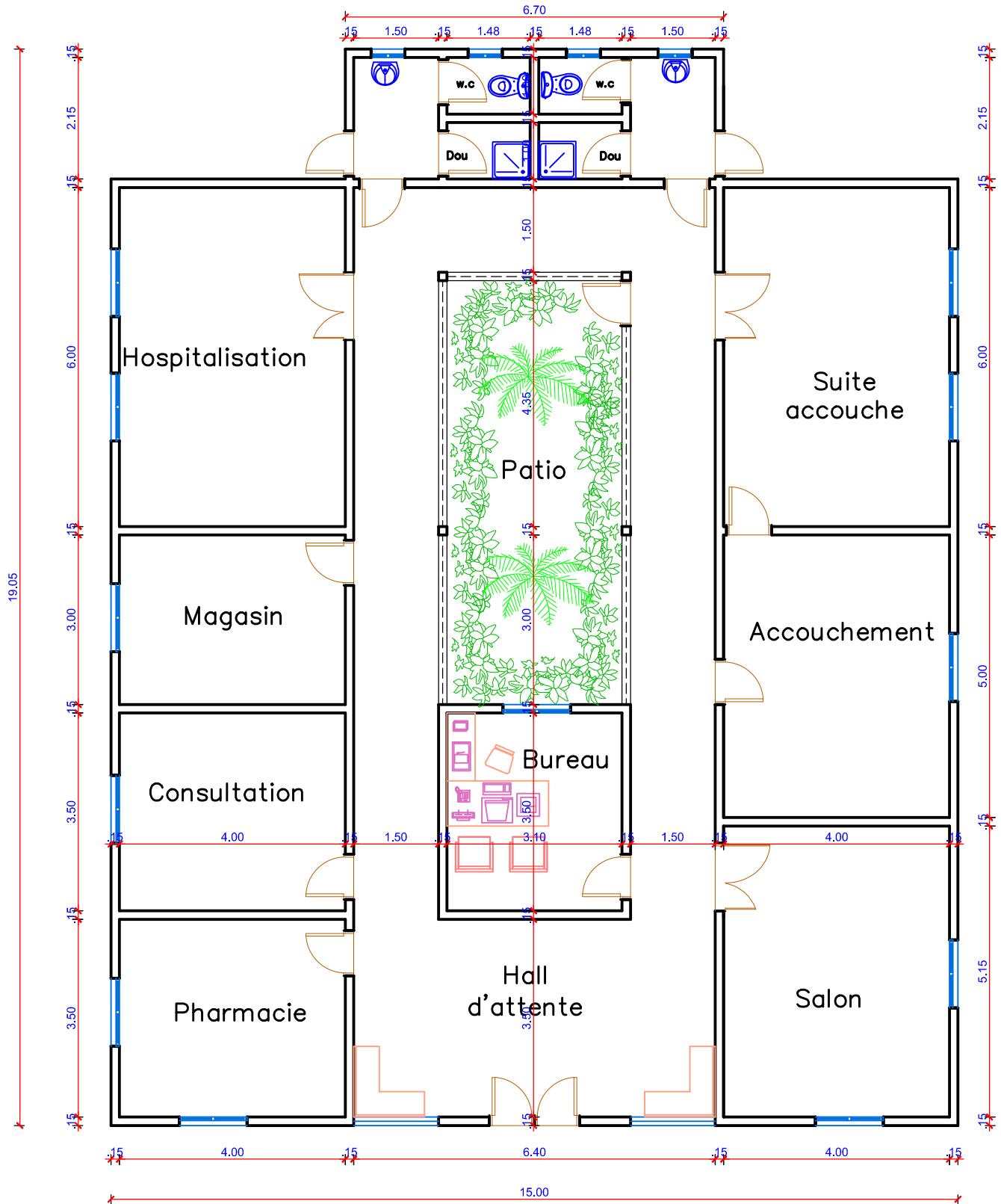
VUE EN PLAN RDC ECHL/1/100
